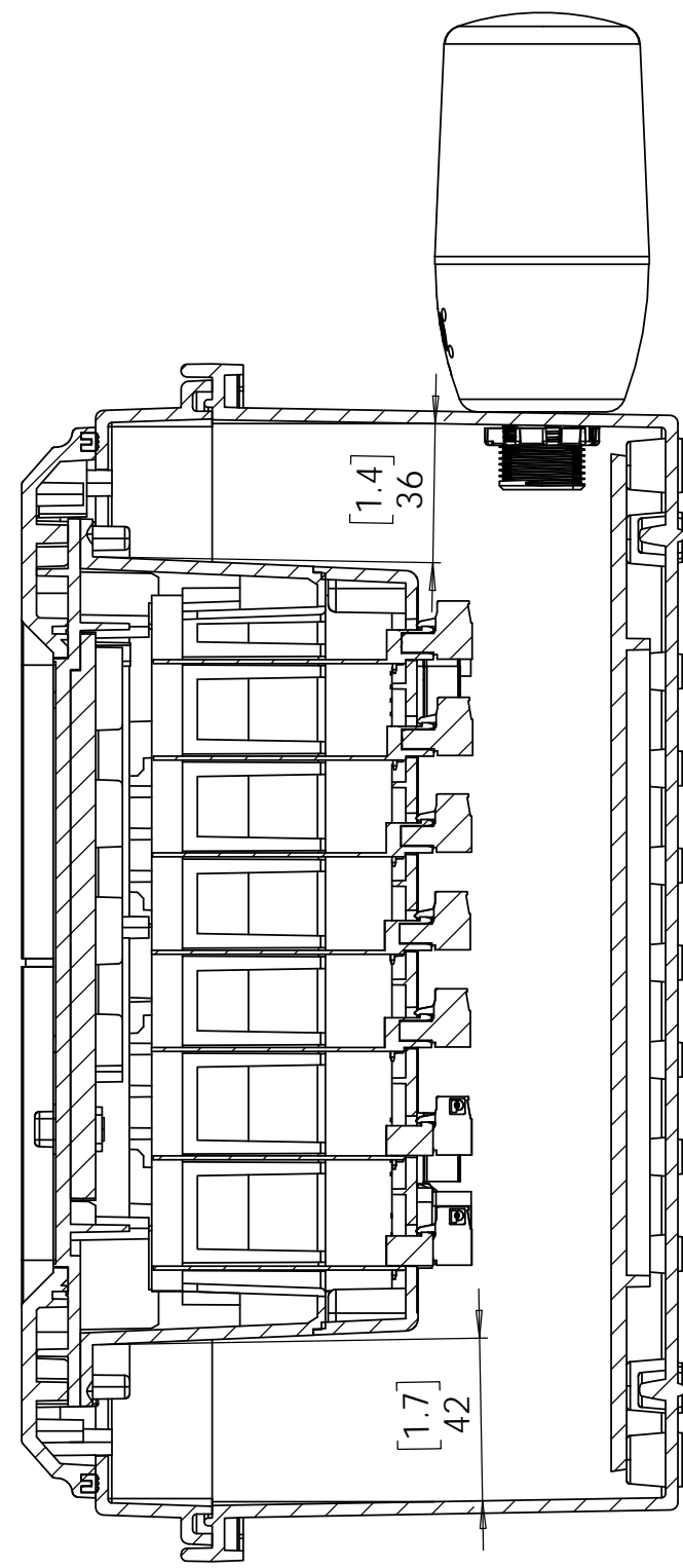
SECTION B-B SCALE 1 : 2
